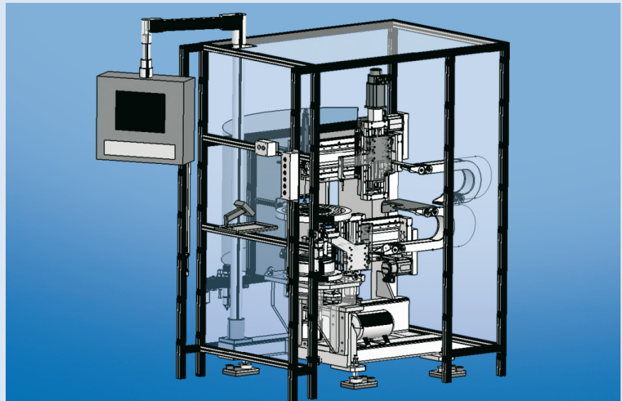
Bild 2: Schutzumhausung (3D-Konstruktion)
