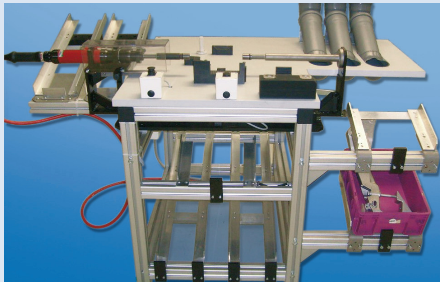
Bild 4: Montagetisch
