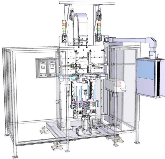
Abb. 1: Gesamtlayout - Federbeinmontage
