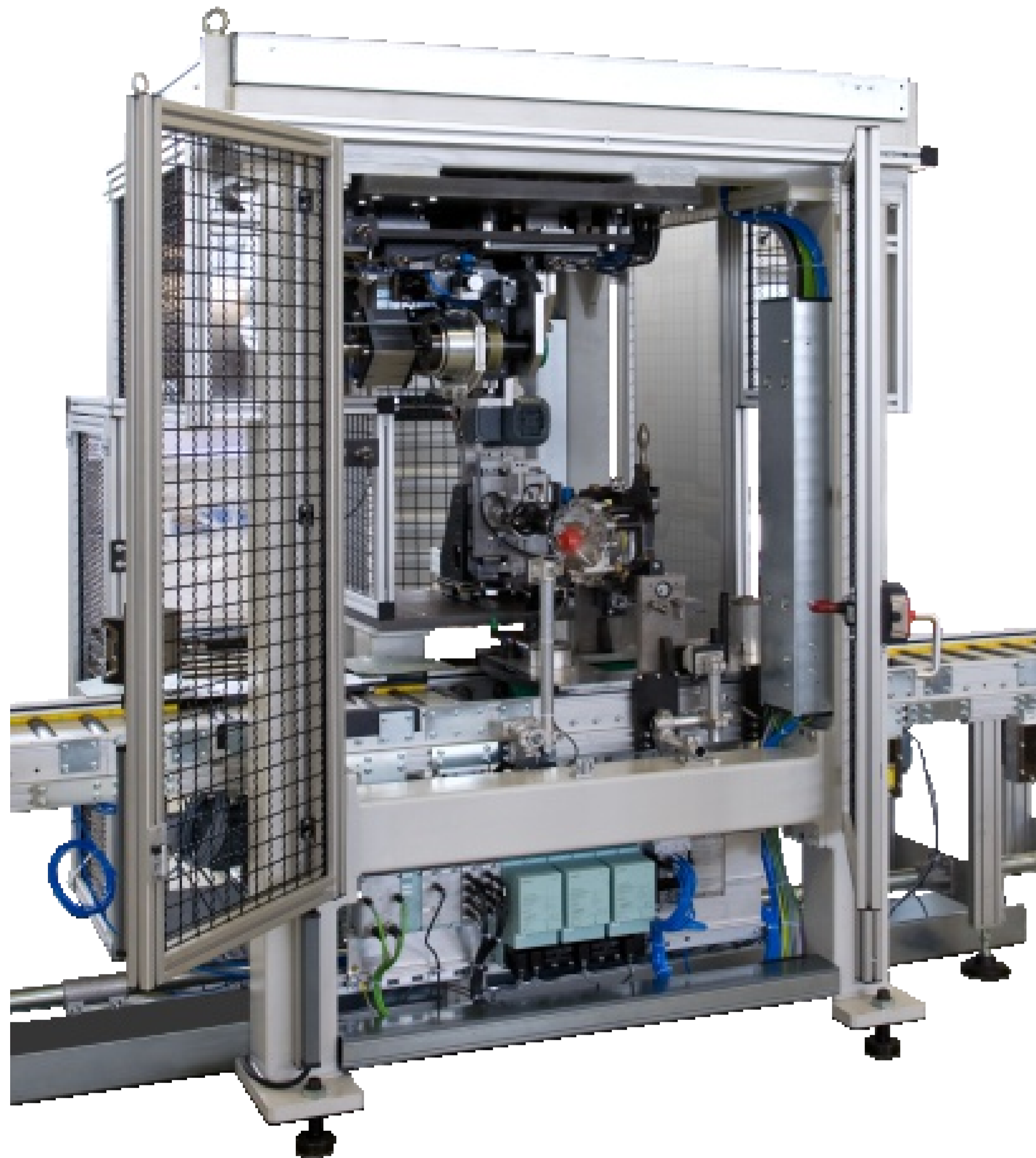
Übersetzungsprüfung Vorderachsgetriebe
